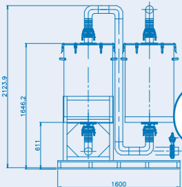
オーダーメイド 製造品の図面(例)
